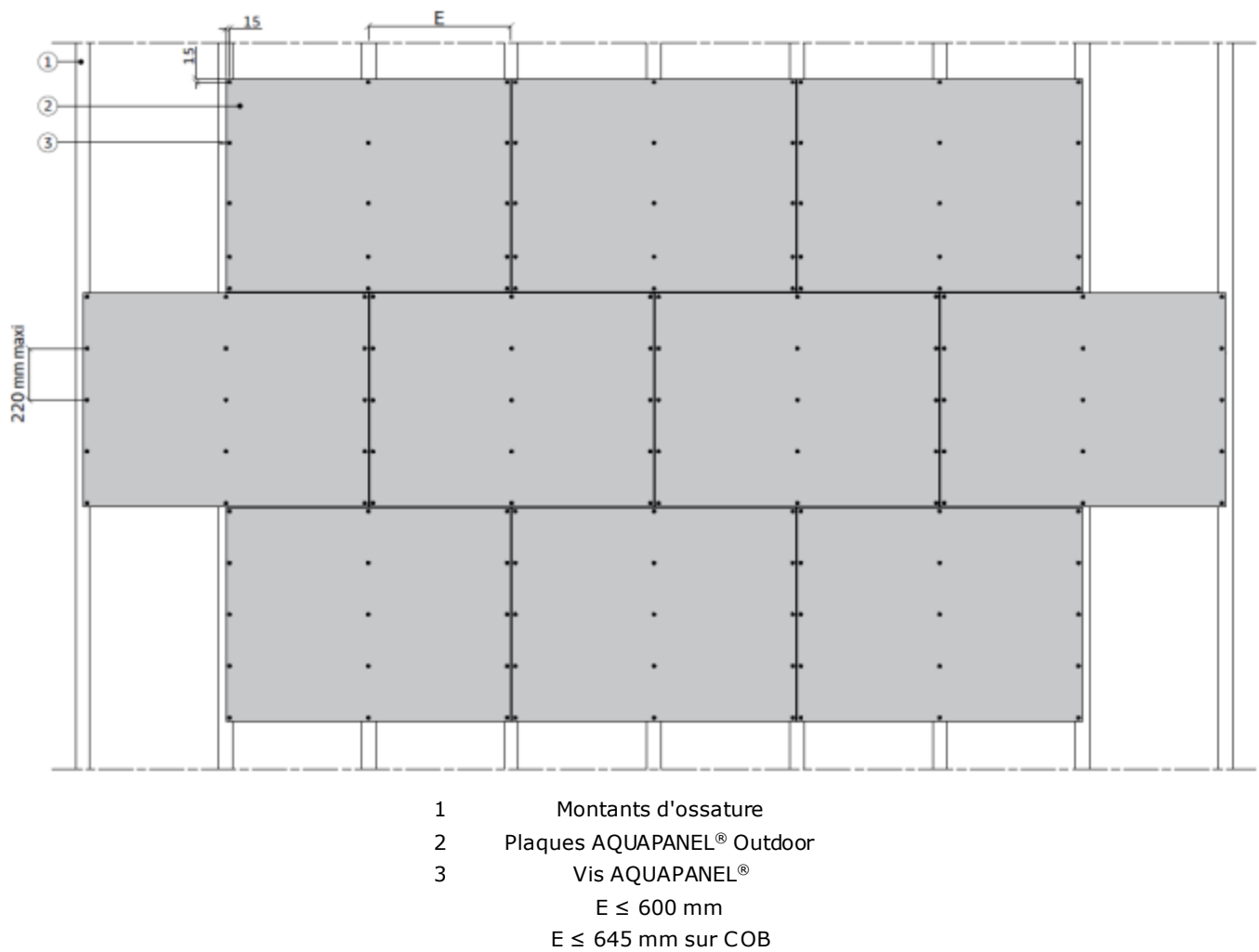
Figure 8 - Calepinage des plaques et espacement des vis - pose horizontale
